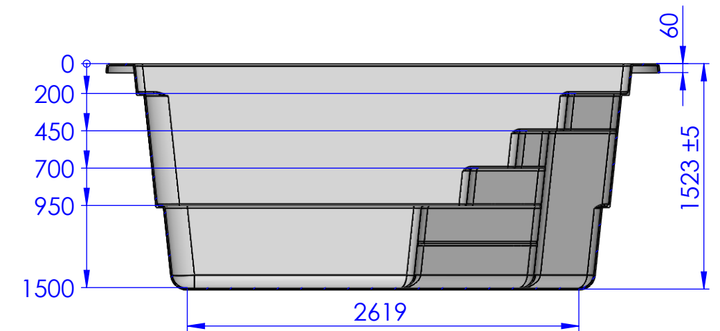
SECTION B-B SCALE 1 : 35
