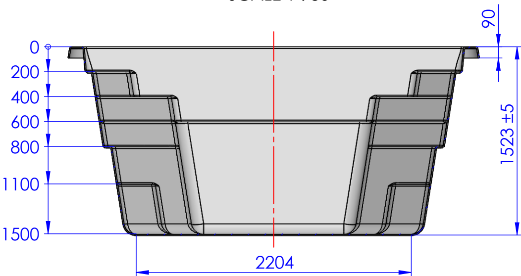
SECTION B-B SCALE 1 : 30
